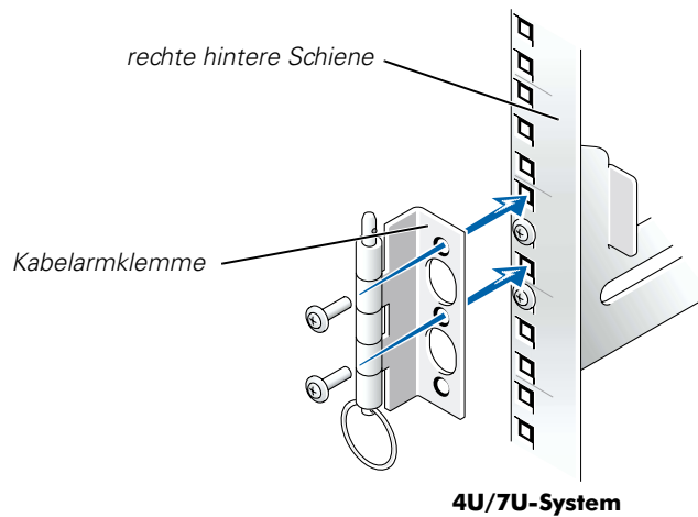
Abbildung 3-4. Befestigung des Kabelarms am Rack
